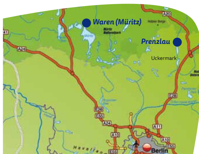
Hier wird, gemeinsam mit der ENERTRAG AG, eine Anlage in Blindow, bei Prenzlau, errichtet. Es handelt sich um eine Vestas V112 mit einer Nabenhöhe von 140 m, einer Nennleistung von 3 MW und einem Rotordurchmesser von 112 m. (Januar 2014)
